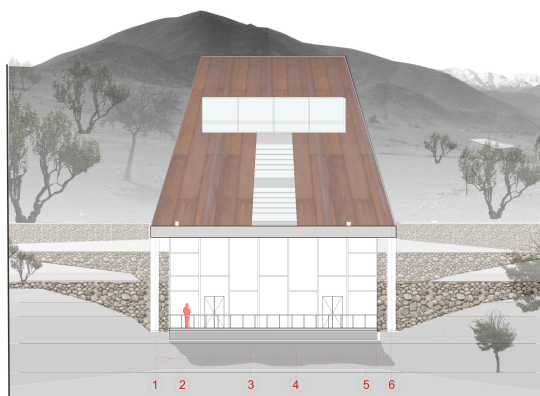
ELEVACION SUR
