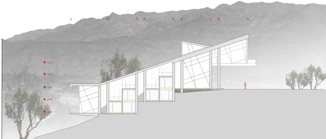
ELEVACION ORIENTE
