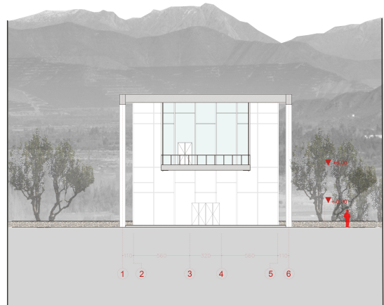
ELEVACION NORTE
