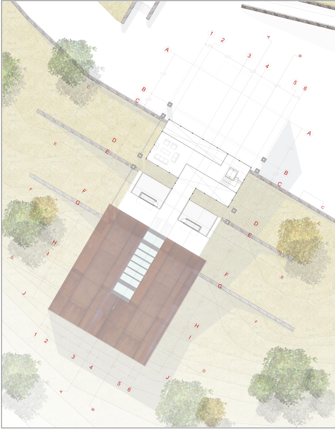
PLANTA NIVEL: +3.00 ESCALA: 1/100
