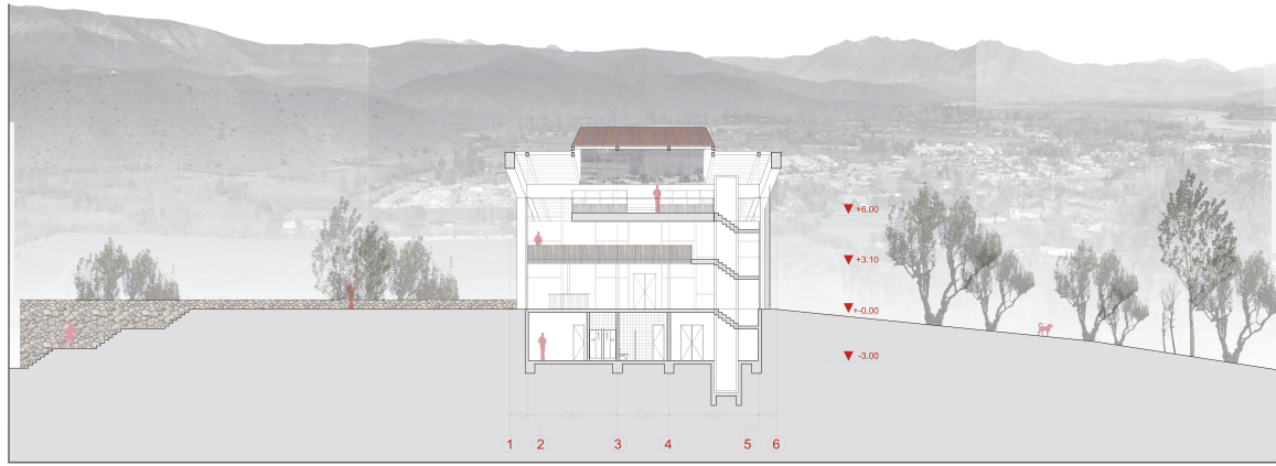
CORTE C-C
