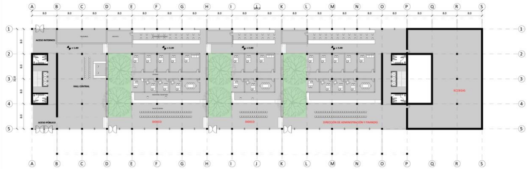
PLANTA PRIMER NIVEL VOLUMEN DIRECCIONES MUNICIPALES
