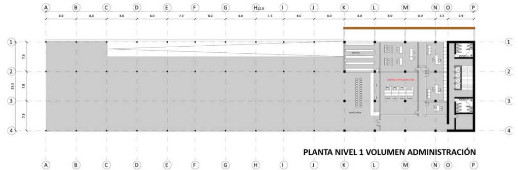
PLANTA NIVEL -1 VOLUMEN ADMINISTRACIÓN
