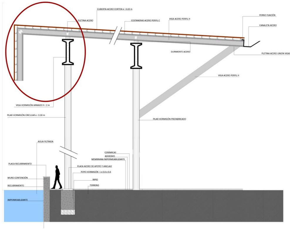
DETALLE CUBIERTA ATRIO
