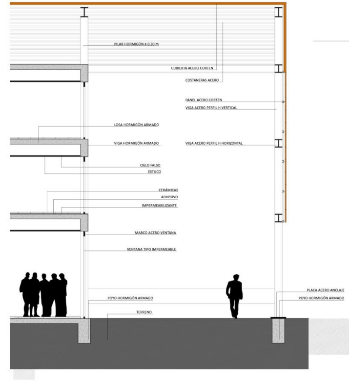
DETALLE CÁSCARA SCREEN-PANEL ACERO CORTEN
