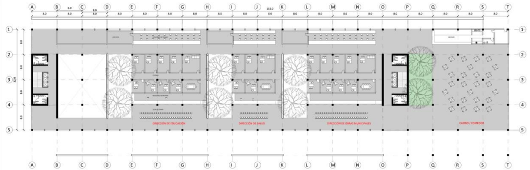
PLANTA SEGUNDO NIVEL VOLUMEN DIRECCIONES MUNICIPALES
