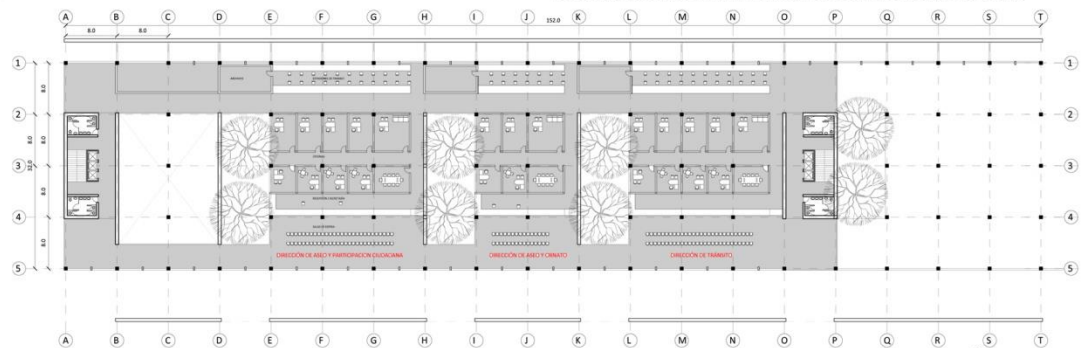
PLANTA TERCER NIVEL VOLUMEN DIRECCIONES MUNICIPALES
