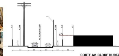
CORTE AV. PADRE HURTADO
