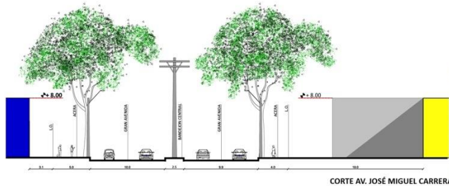
CORTE AV. JOSÉ MIGUEL CARRERA
