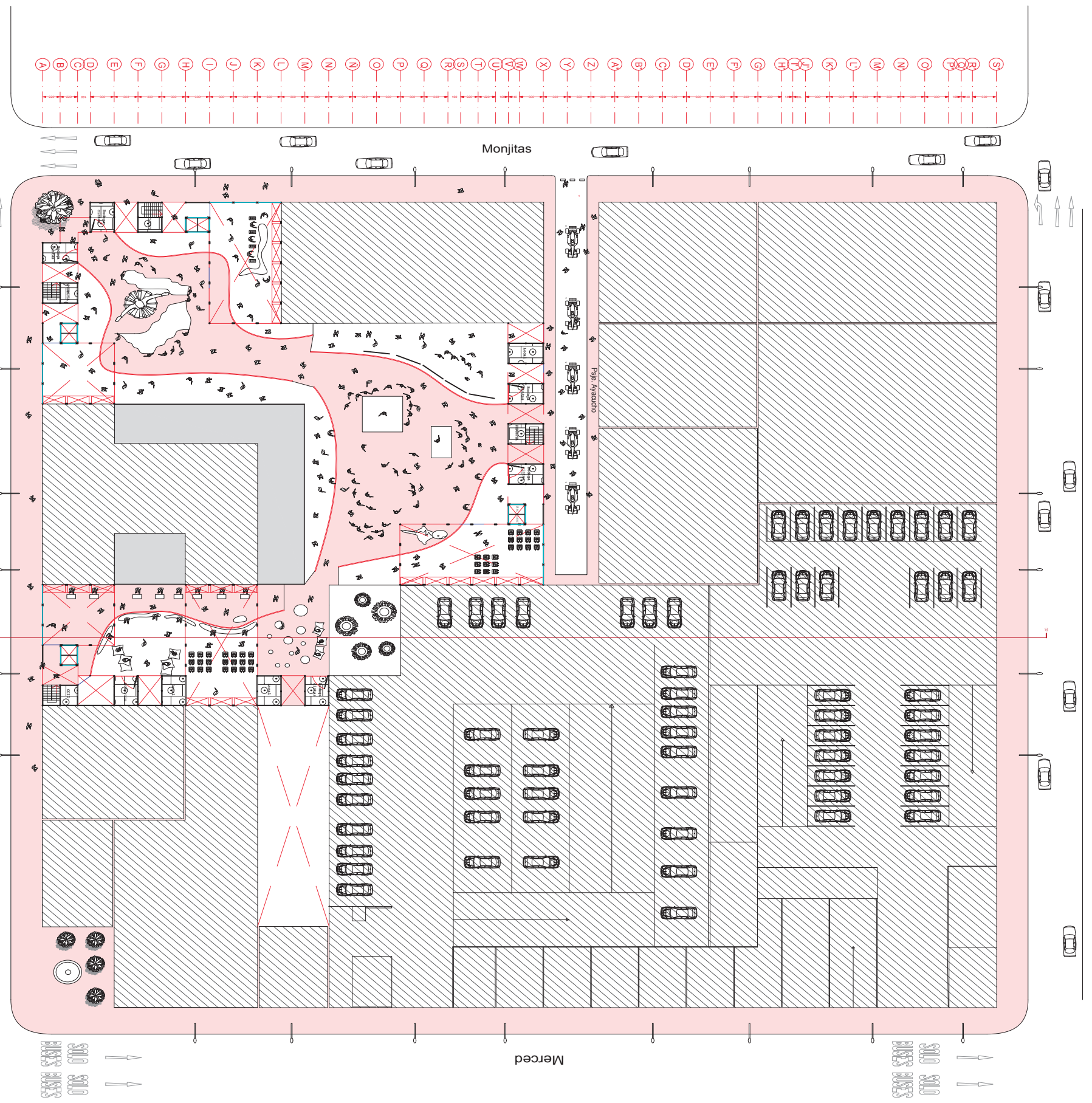
PLANTA NIVEL CALLE COLECTIVO - PUBLICO ESCALA 1:200 Intercambio permutacion interaccion mutualidad Adicion
